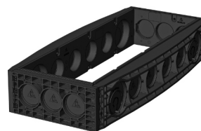
Rama 220 mm Nr produktu: BP-102384 3 x Ø 110 6 x Ø 110 / 2 x Ø 160 Waga: 23,0 kg
