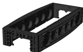
Rama 220 mm Nr produktu: BP-102389 1 x prostokąt 6 x Ø 110 / 2 x Ø 160 Waga: 22,0 kg
