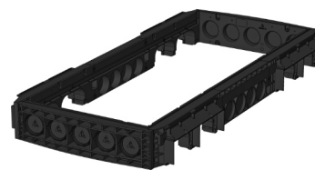
Rama 220 mm Nr produktu: na zapytanie 5 x Ø 110 4 x prostokąt / 4 x Ø 110 Waga: 65,5 kg
