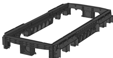
Rama 220 mm Nr produktu: na zapytanie 2 x prostokąt / 1 x Ø 110 4 x prostokąt / 4 x Ø 110 Waga: 59,0 kg
