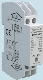
DS98L-400 SPD Typ 2+3 zum Schutz der Ladestation
